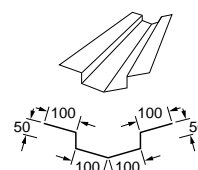
Försänkt rännedal L=2000 mm
