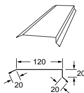
Rännedal L=2000 mm
