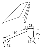
Nockplåt tegelprofil L=2250 mm Täckande L=2140 mm
