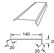
Försänkt rännedal L=2000 mm
