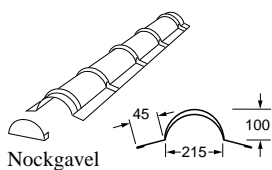
Nockplåt tegelprofil L=2250 mm Täckande L=2140 mm
