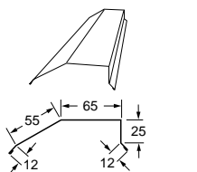
Nockplåt tegelprofil L=2250 mm Täckande L=2140 mm
